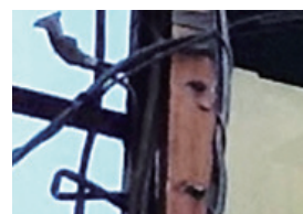
鉄骨接合部（ボルト、ナット、 ビス）のゆるみ、欠落
