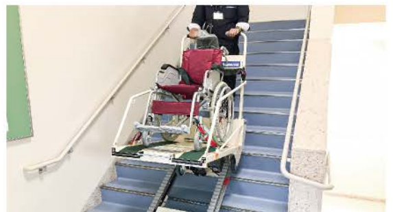
C 小中学校に設置した階段昇降車
