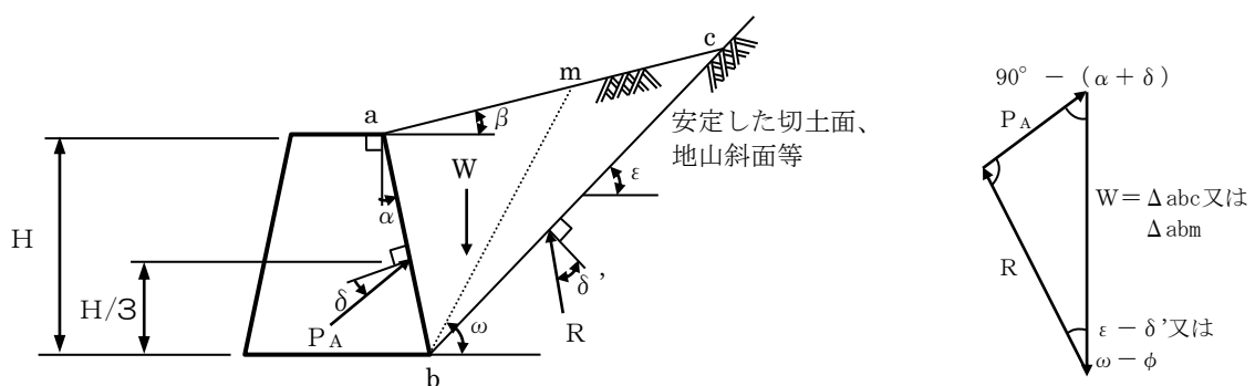
図 5－27 切土部土圧の算定（1）
